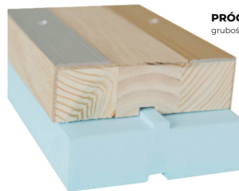
WKŁADKA TERMICZNA POD PRÓG DREWNIANY
