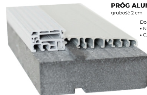
WKŁADKA TERMICZNA POD PRÓG ALUMINIOWY
